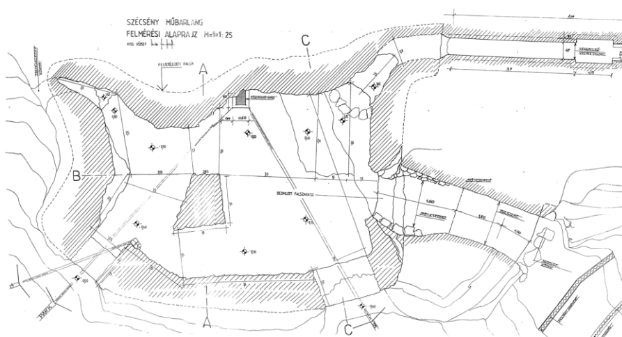
11. ábra A műbarlang felmérési rajza (K. J.)
